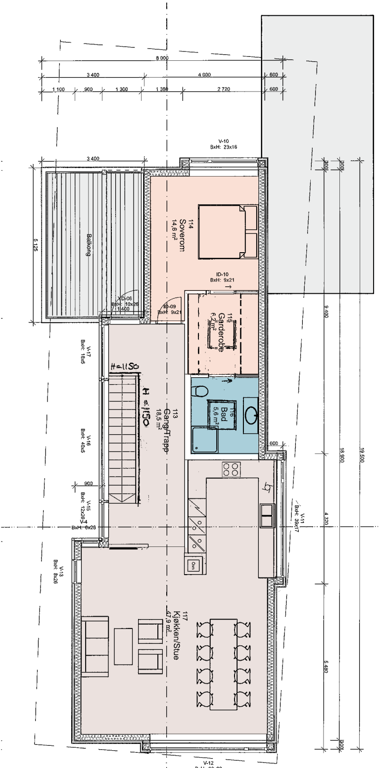
Plan 2. etasje / Hovedstue / Kjøkken Master soverom / Garderobe / Bad
