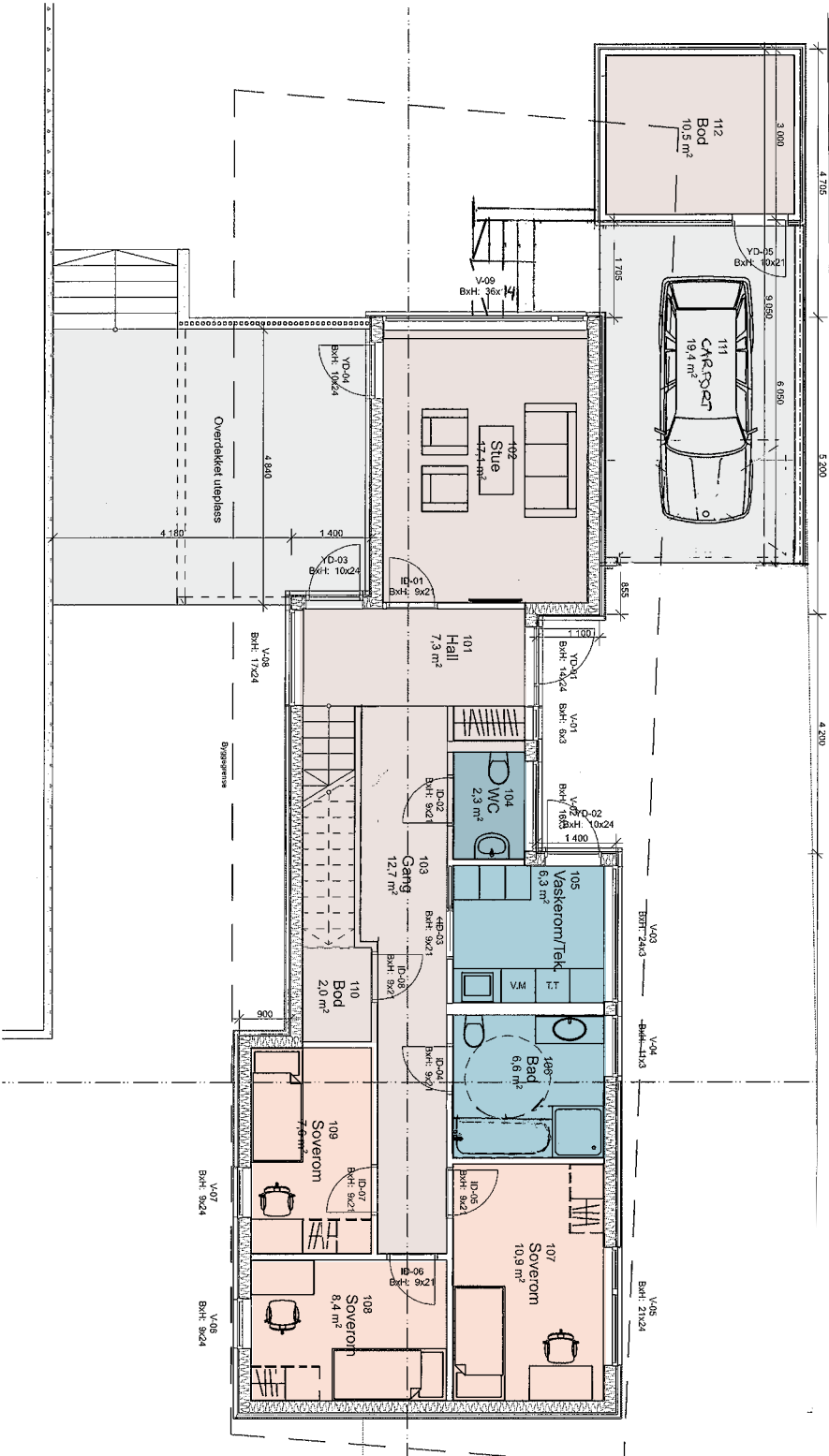
Plan 1. etasje / 3 sov / TV-stue Bad / WC / Vaskerom / Bod / Carport
