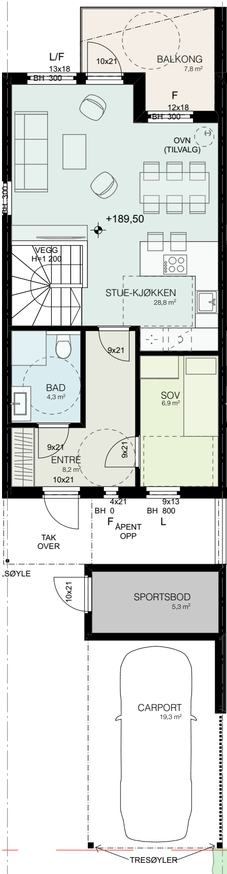
1.etg
